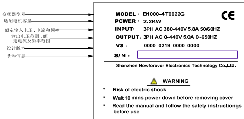
图 1-2 B1000 变频器铭牌
